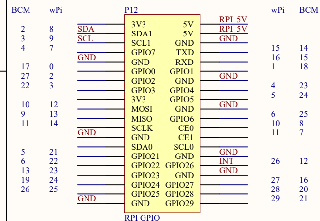
RPI GPIO
